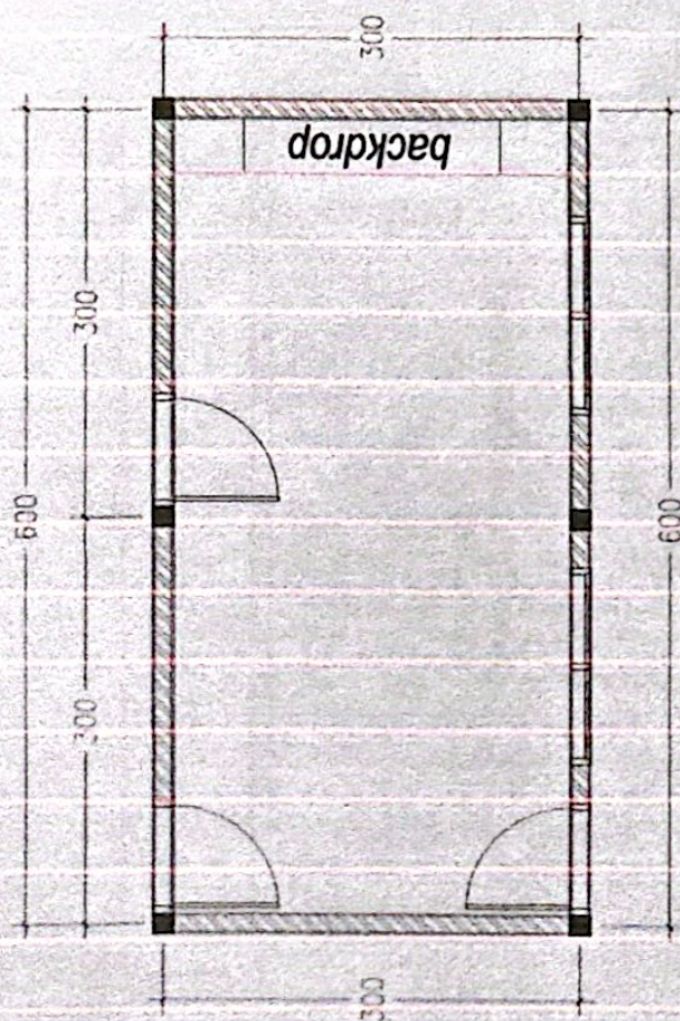
DENAH RENCANA Skala 1 : 50
